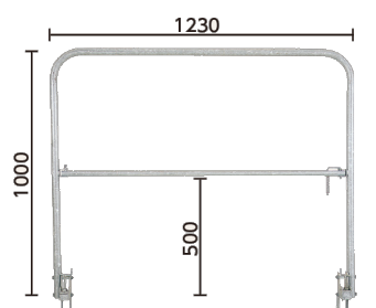
●簡易手すり(長)5.2kg
